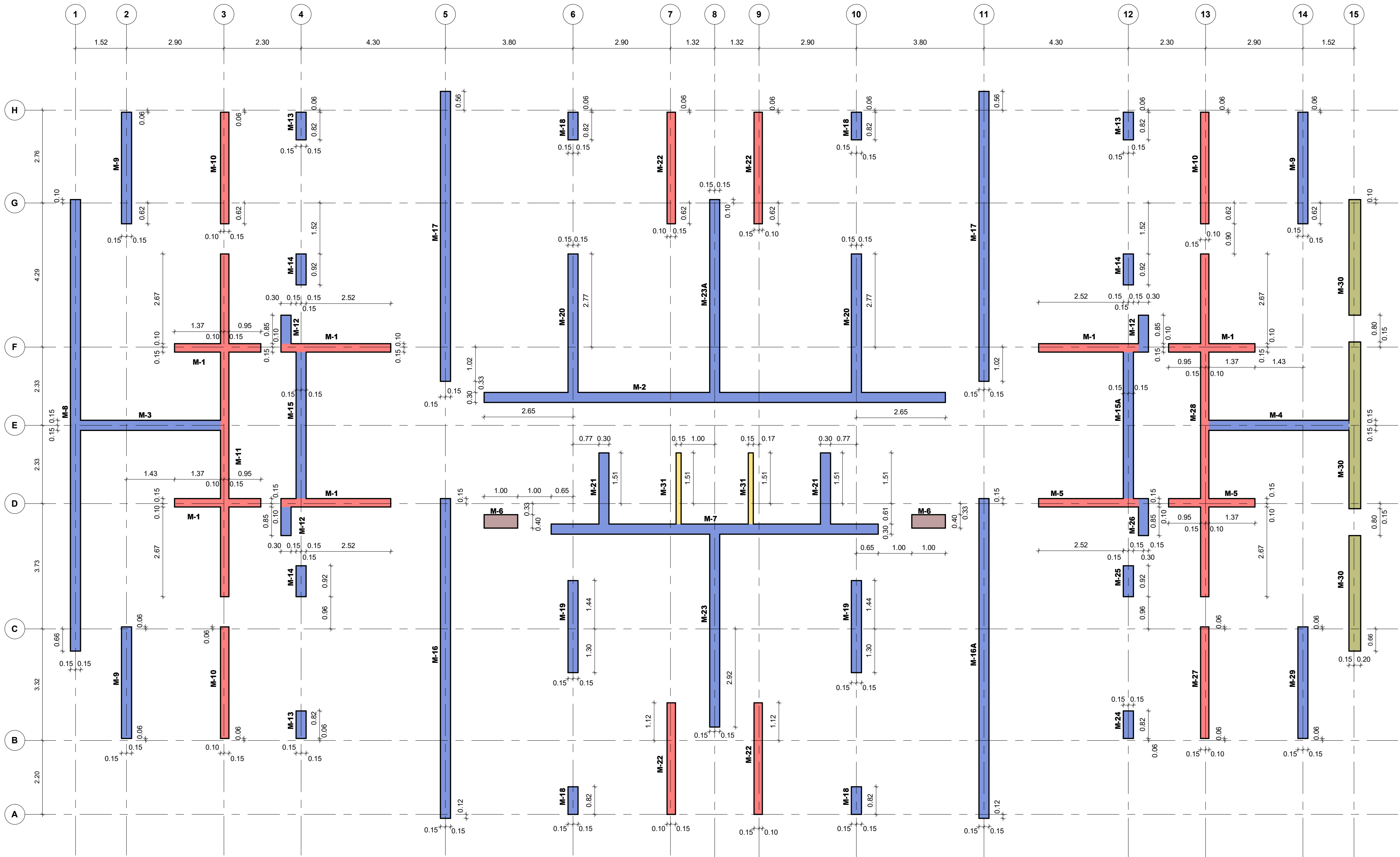
PLANTA LOCALIZACIÓN DE MUROS PISO TIPO 2 ( PISO 15 A PISO 21 ) Escala 1 : 75
